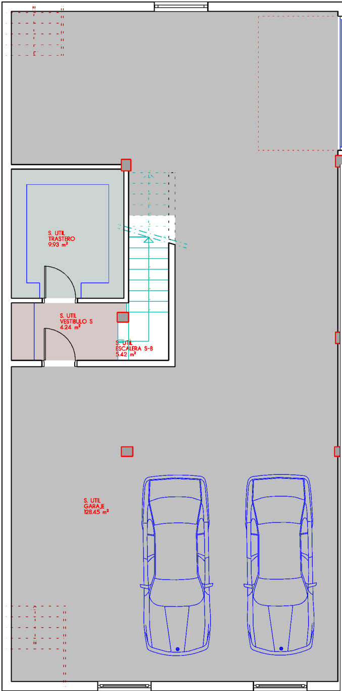
PLANTA SOTANO PROYECTO
